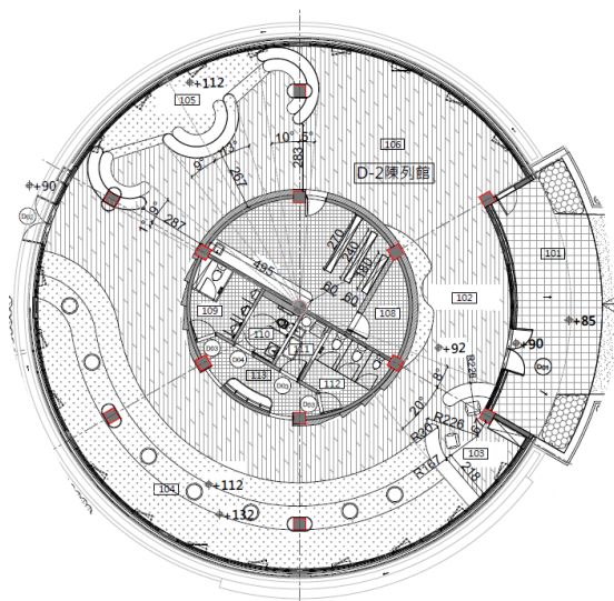
圖 10 親子環教生態館配置圖
