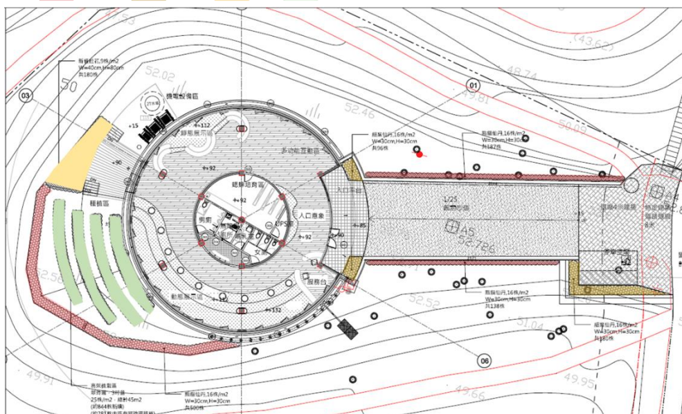
圖11 植栽配置圖
