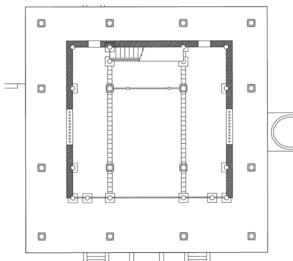
文昌閣一樓平面圖
