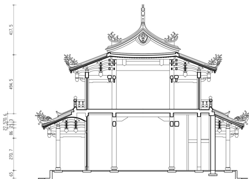
圖 7 海神廟剖立面圖
