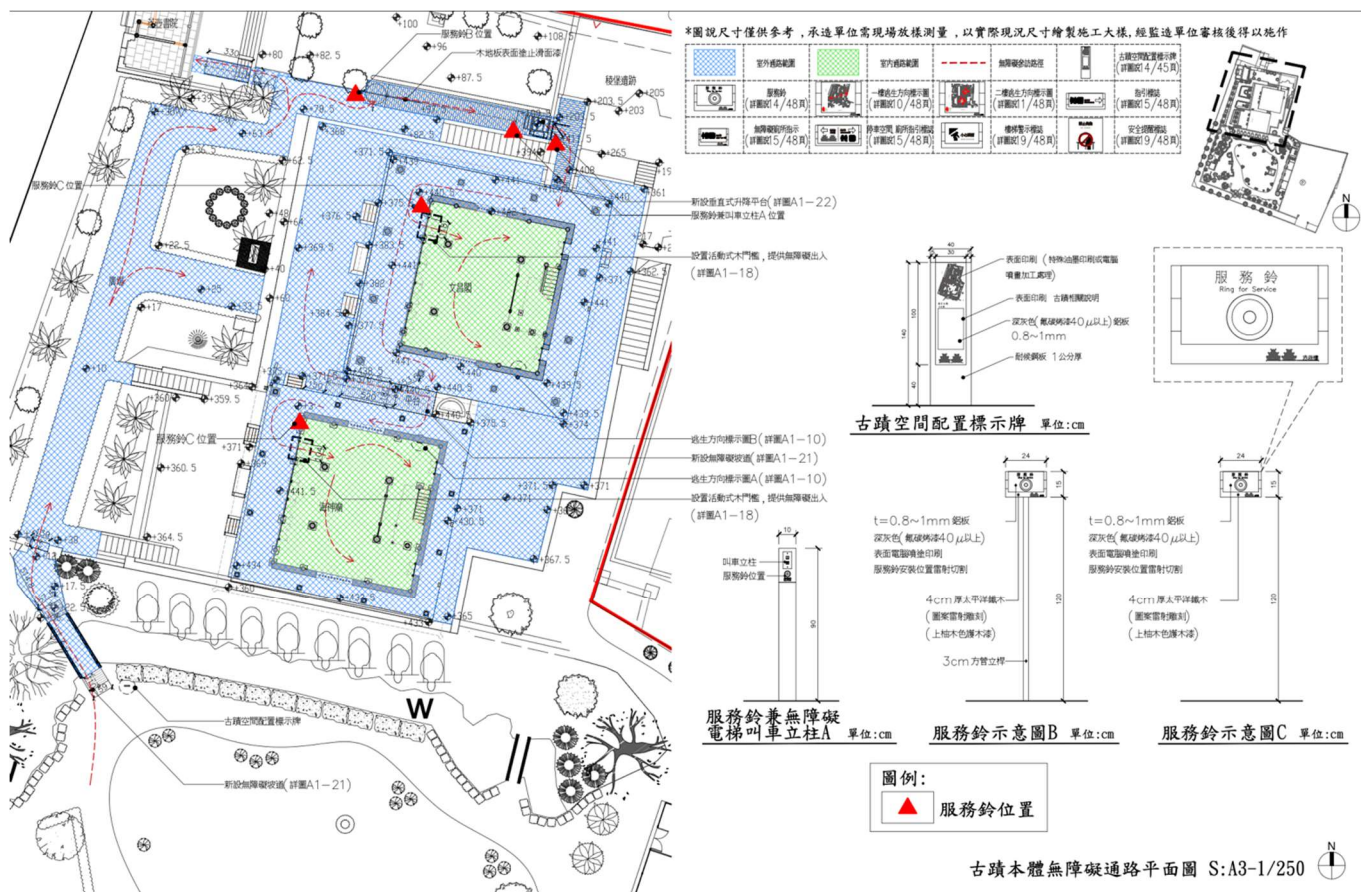
圖 14 無障礙設施平面配置圖
