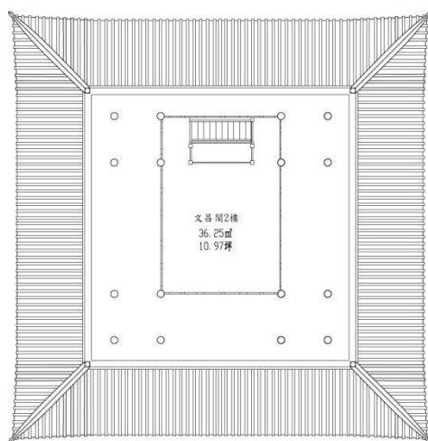
文昌閣二樓平面圖
