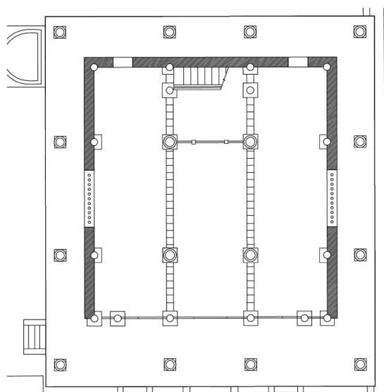
海神廟一樓平面圖
