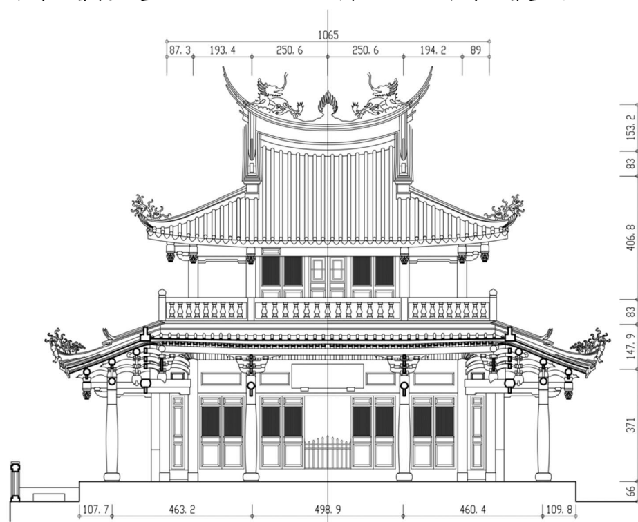
圖3 文昌閣剖立面圖
