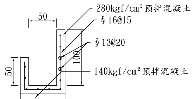
施工斷面圖
