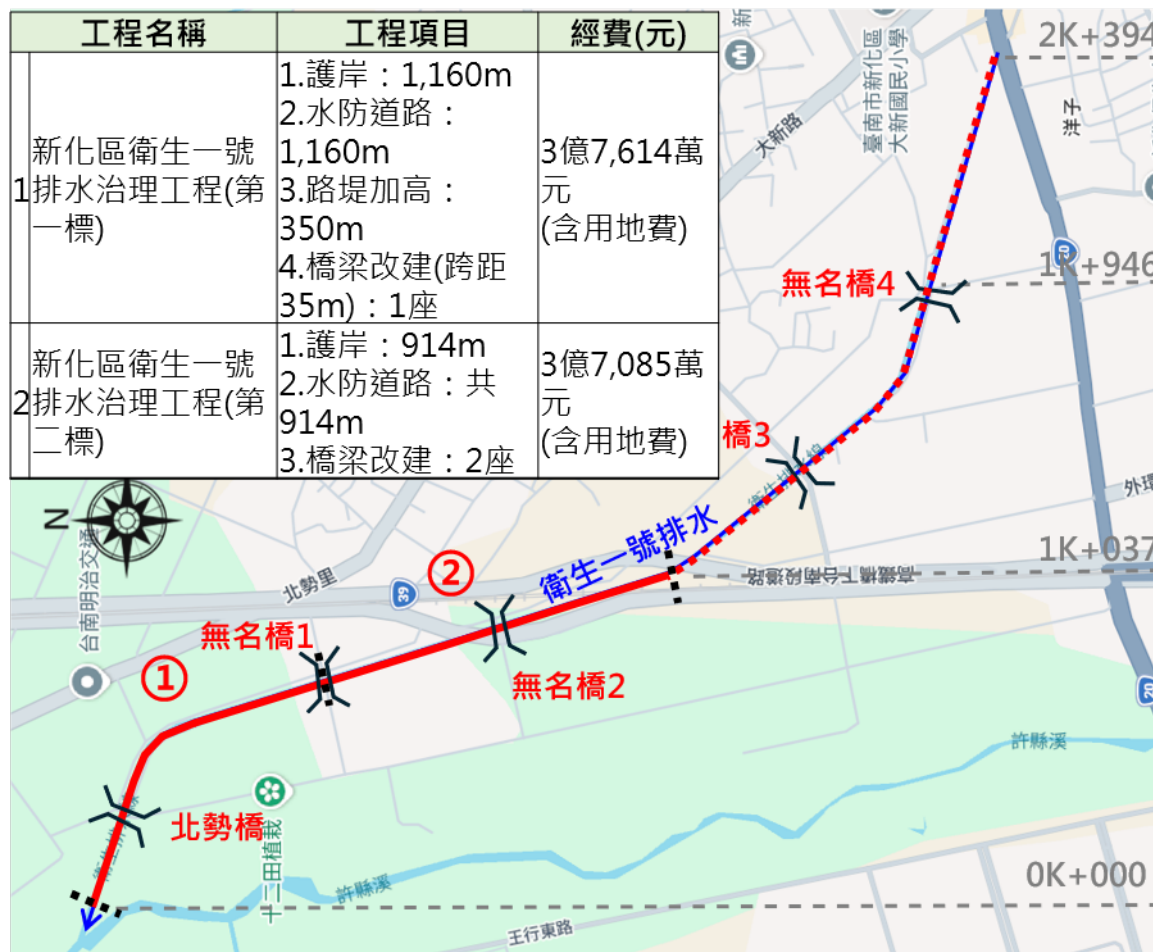
工程位置圖
