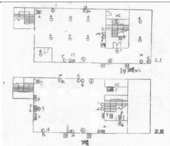
3F、屋頂平面圖
