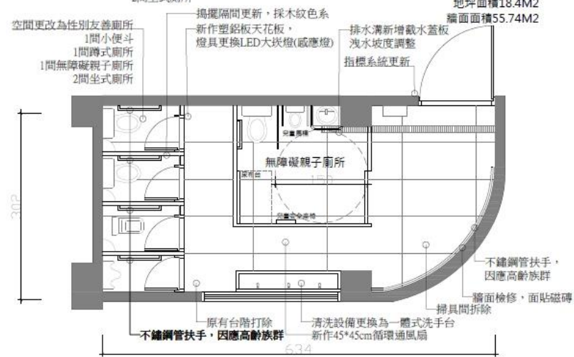
右側性別友善及無障礙親子廁所平面圖 S=1/50(A3) 地坪面積18.4M2 牆面面積55.74M2
