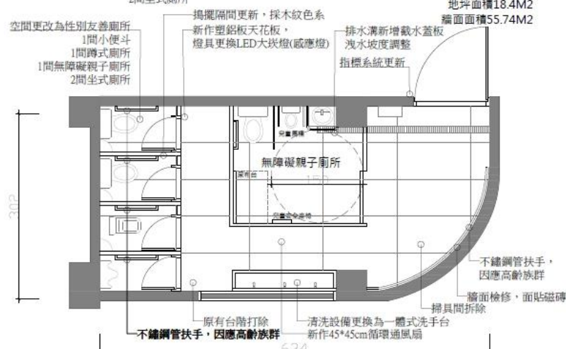
右側性別友善及無障礙親子廁所平面圖 S=1/50(A3) 地坪面積18.4M2 牆面面積55.74M2
