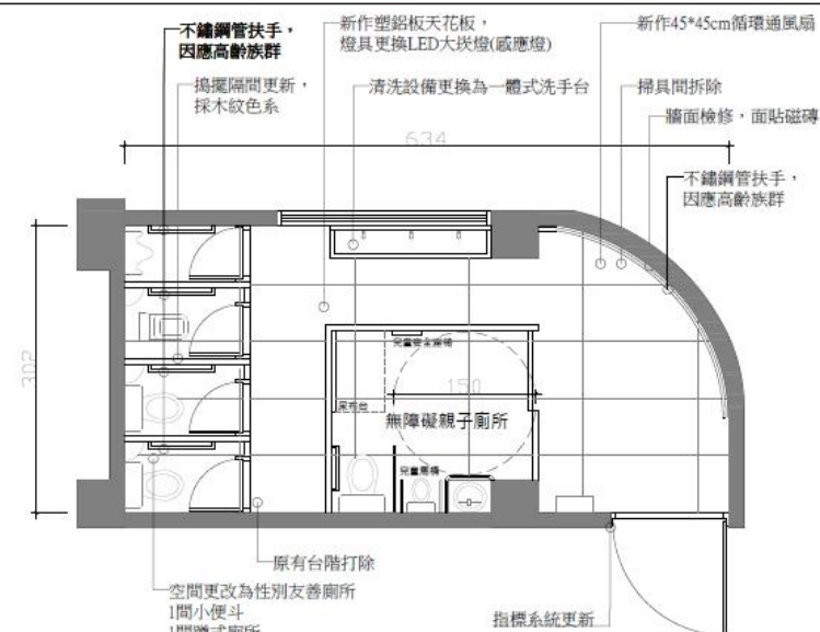
左側性別友善及無障礙親子廁所平面圖 (S=1/500(A3)) 地坪面積18.4M2 牆面面積55.74M2
