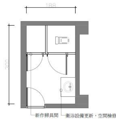
左後廁所平面圖 (S=1/50(A3)) 地坪面積5.64M2 牆面面積29.28M2
