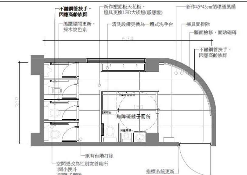
左側性別友善及無障礙親子廁所平面圖 (S=1/50(A3)) 地坪面積18.4M2 牆面面積55.74M2
