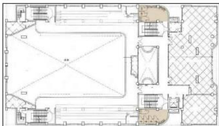
四層平面圖
