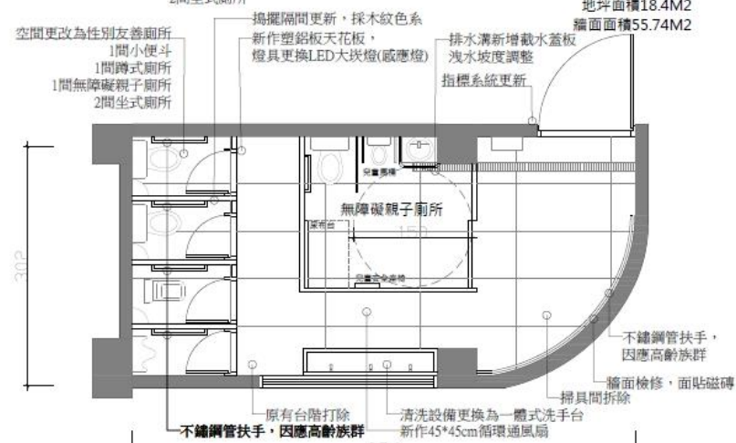
右側性別友善及無障礙親子廁所平面圖 (S=1/500(A3)) 地坪面積18.4M2 牆面面積55.74M2
