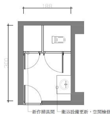
左後廁所平面圖 S=1/50(A3) 地坪面積5.64M2 牆面面積29.28M2
