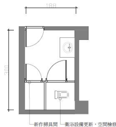
右後廁所平面圖 S=1/50(A3) 地坪面積5.64M2 牆面面積29.28M2
