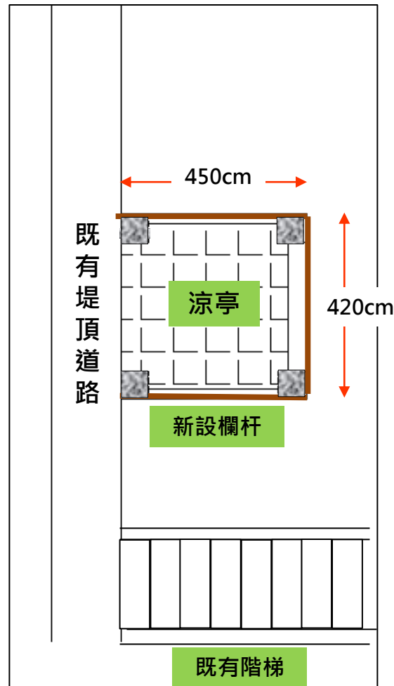
配置平面圖
