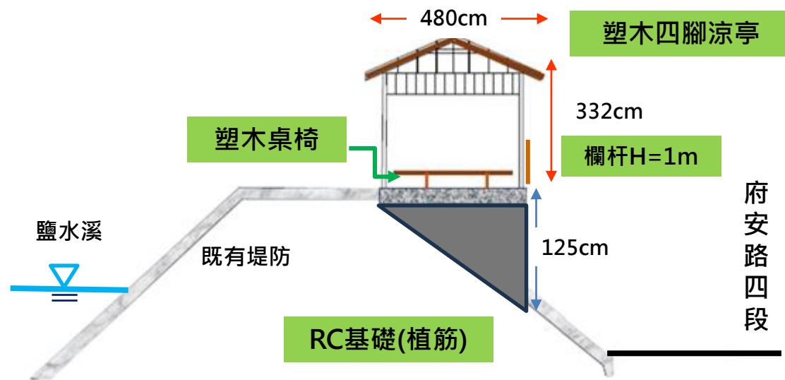
堤頂增設涼亭標準圖
