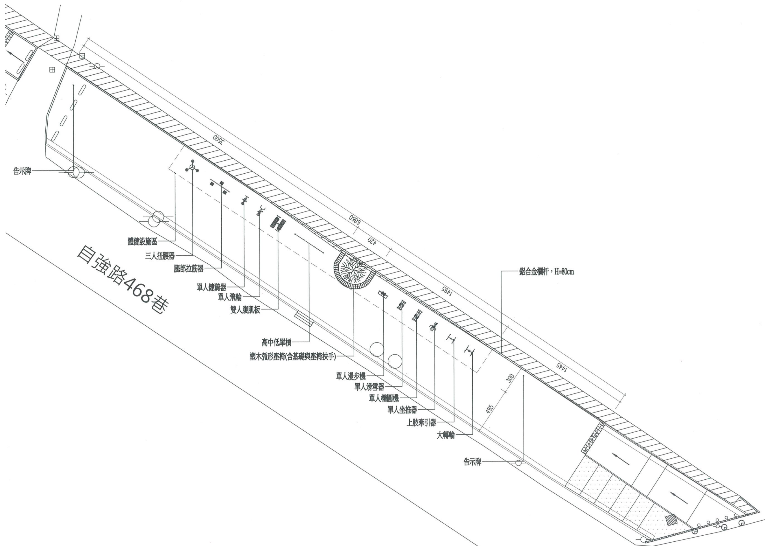
埔園里自強路468巷旁人行步道設置體健設施平面圖
