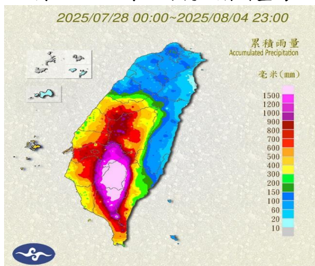
圖 1 7 月 28 日 00 時至 8 月 4 日 23 時西南氣流期間臺灣全島累積雨量圖
