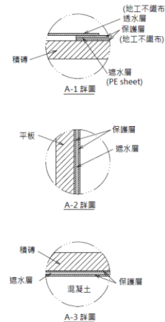
貯留型槽磚結構外層示意圖
