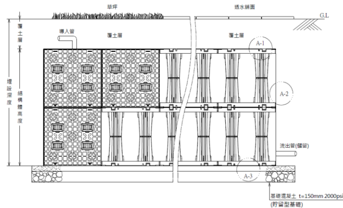
槽磚式雨水貯留結構示意圖
